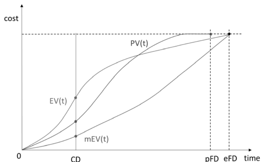
Рис. 6. Кривые EV(t), PV(t) и mEV(t) с учетом прогноза до конца проекта.
